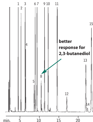
Rt-CW20M™ F&F column
